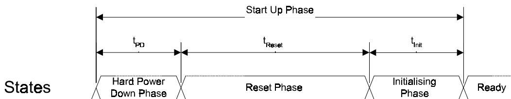
图 11-1 启动过程
