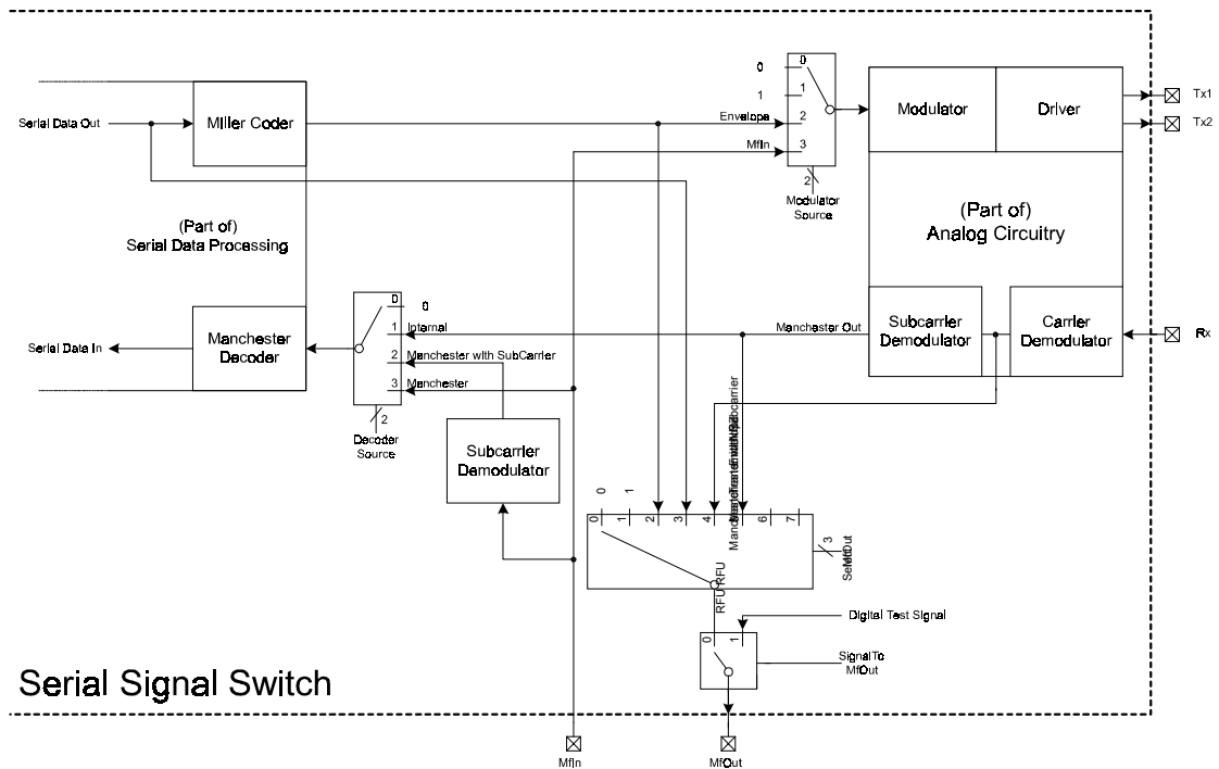
图 15-1 串行数据转换
