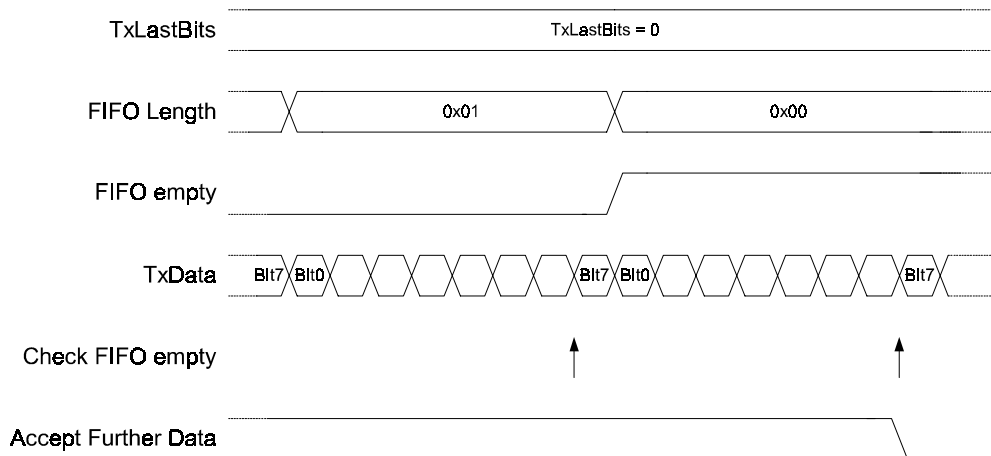
图 16-2 字节方式帧的发送时序
