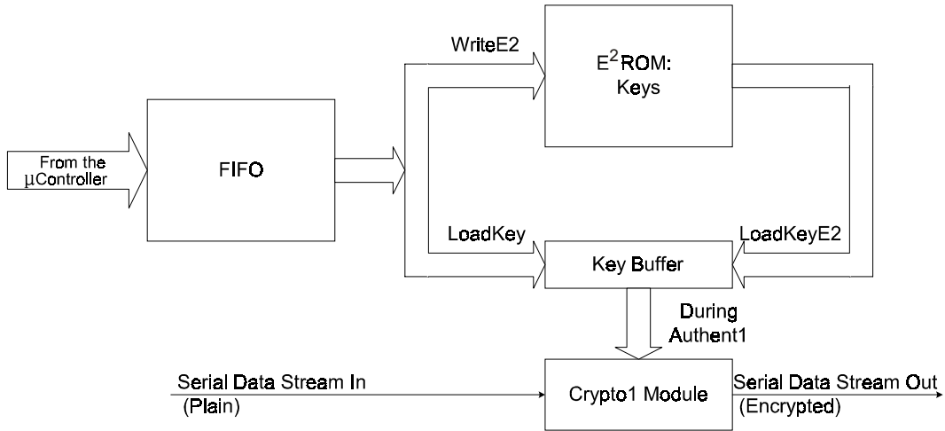
图 17-1 密匙处理: 方框图
